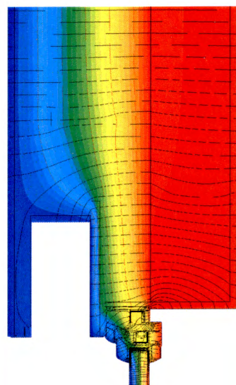
Isothermenbild
